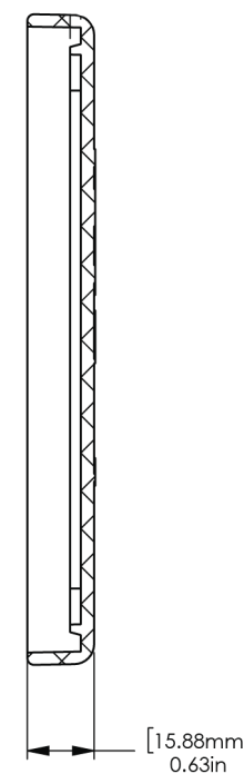
SECTION D-D
